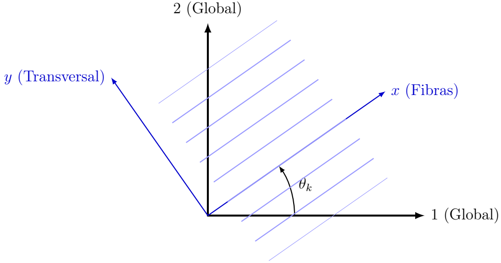
Figura 8.2: Orientação estrutural da lâmina k . O ângulo \theta_k define a rotação do sistema local ortotrópico (x, y) em relação ao referencial macroscópico global do laminado (1, 2) .
